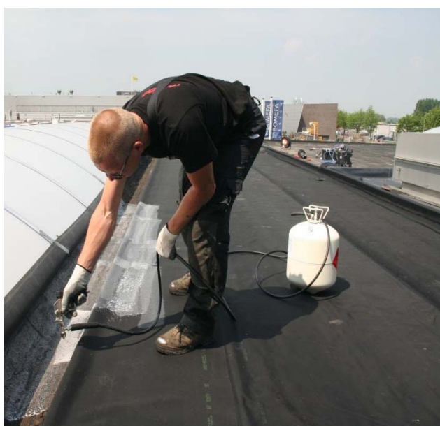
Figure 2 – Collage du relevé à la colle HERTALAN KS 205 (pulvérisation de la colle)
