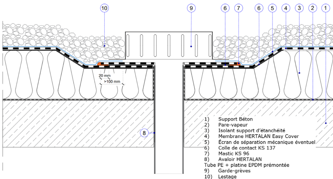
Figure 12 – Évacuation d'eaux pluviales
