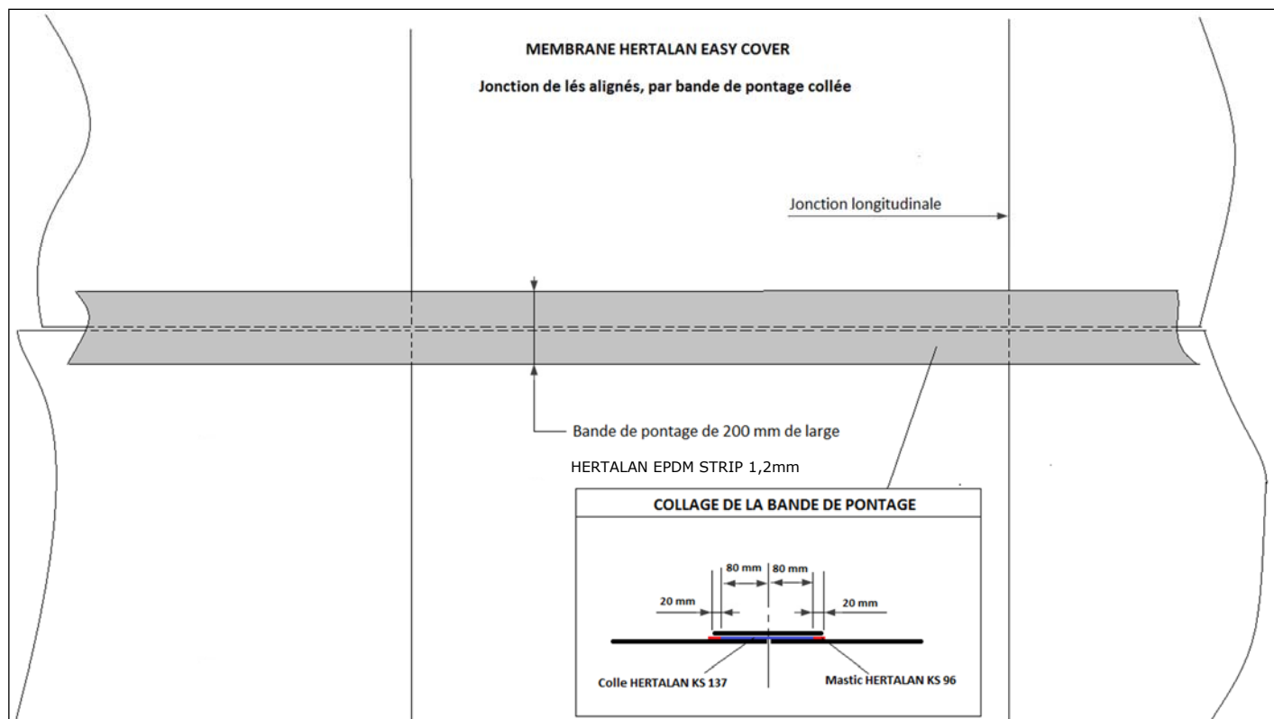
Figure 4 - HERTALAN Easy Cover, joints alignés avec bande de pontage collée
